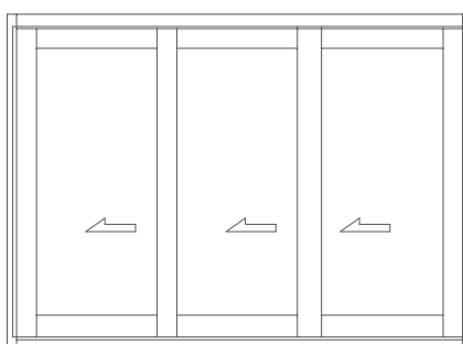
Cửa đi lùa 03 cánh
