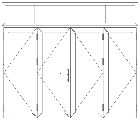
Cửa đi 04 cánh - Fix rời
