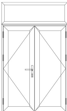
Cửa đi 02 cánh Fix rời
