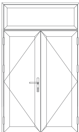
Cửa đi 02 cánh Fix liền
