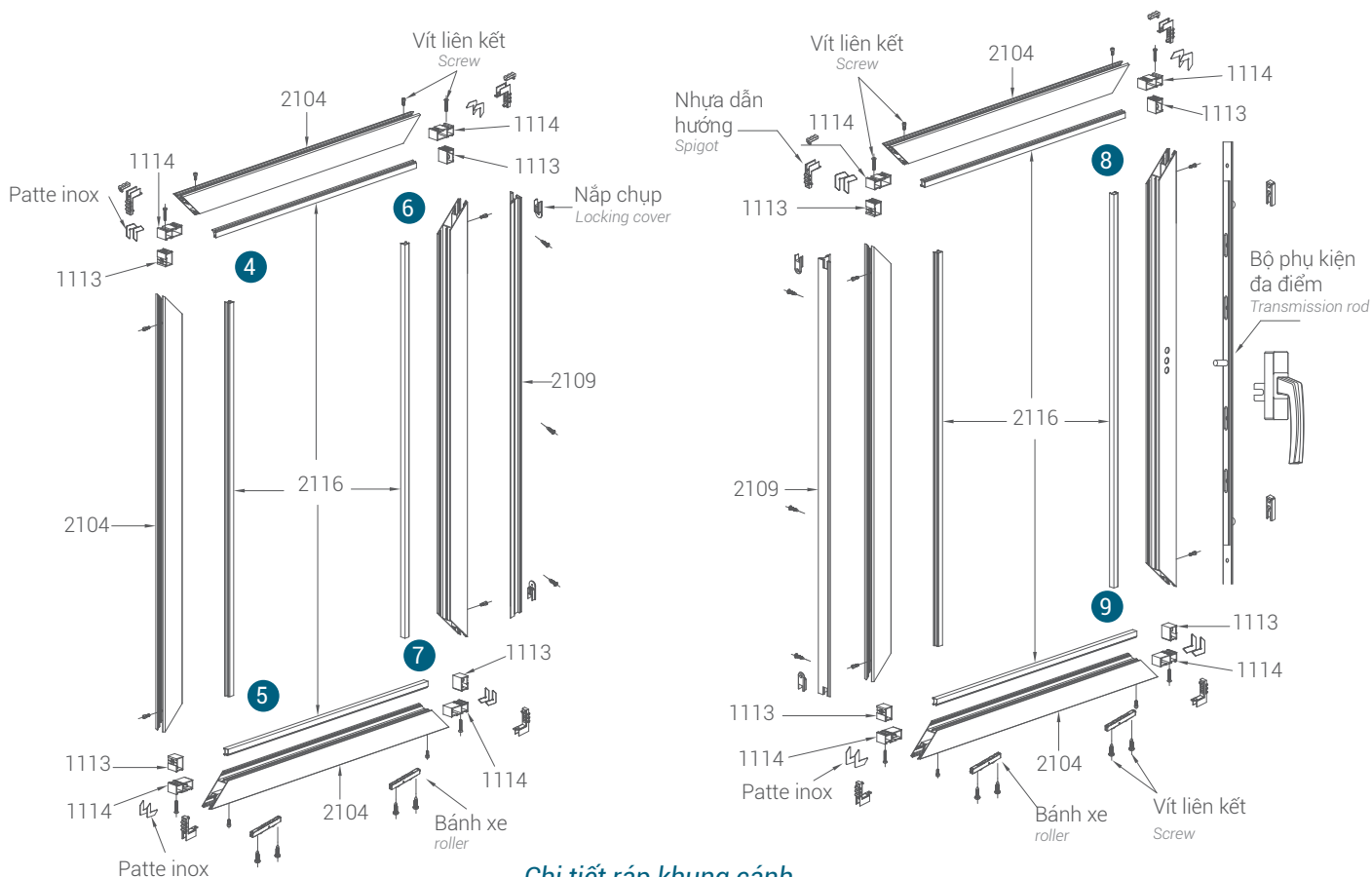
Chi tiết ráp khung cánh Leaf frame details
