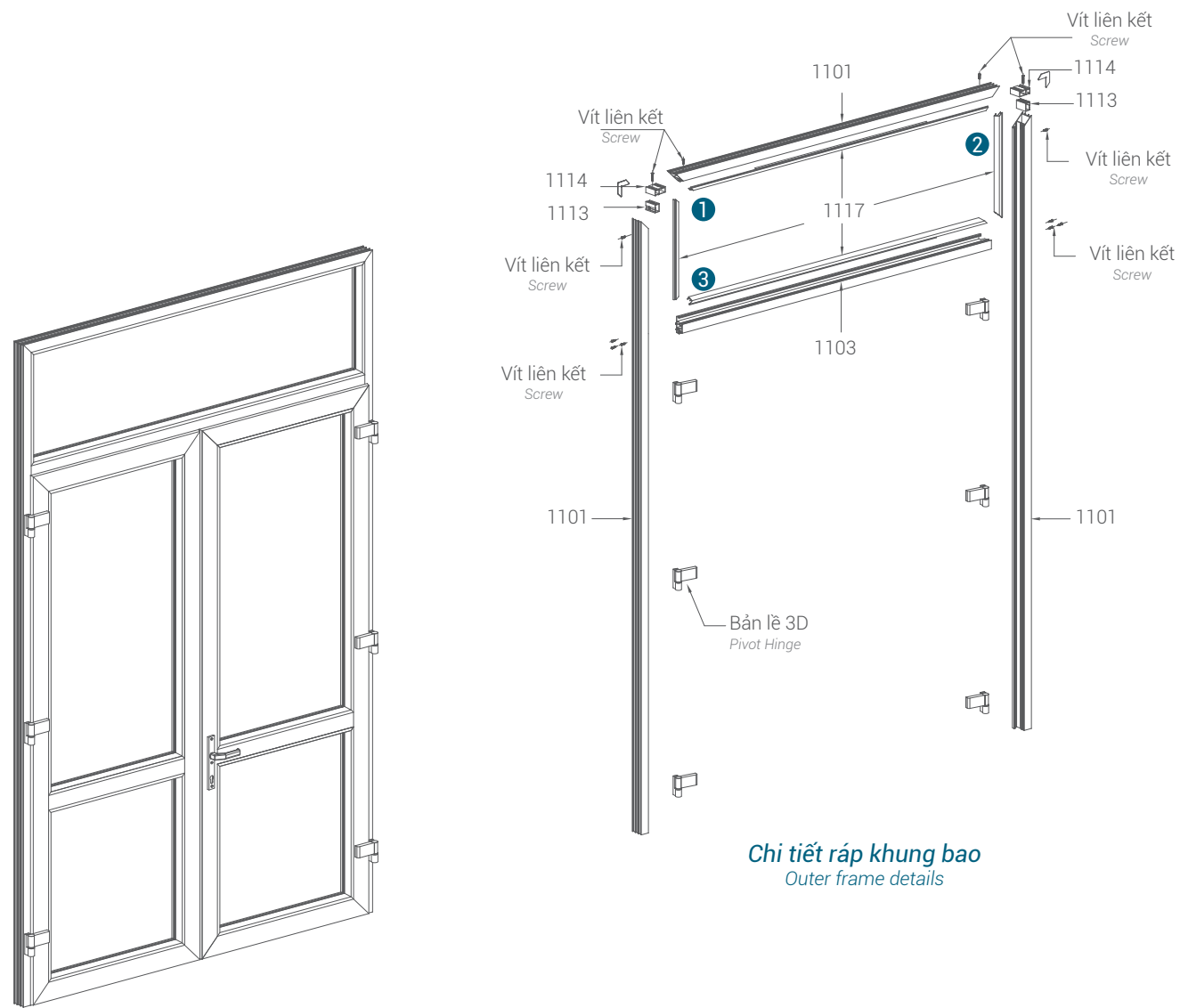
Lắp ráp hoàn thiện Complete assembly diagram
