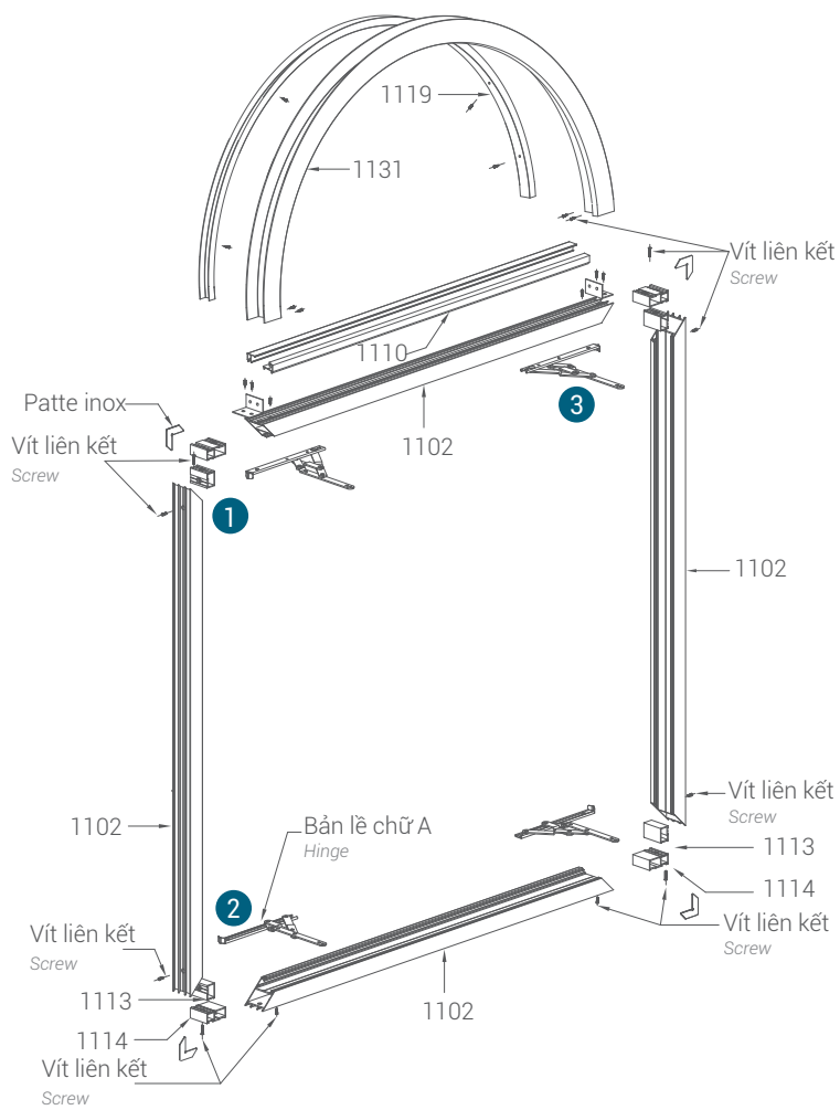
Chi tiết ráp khung bao Outer frame details
