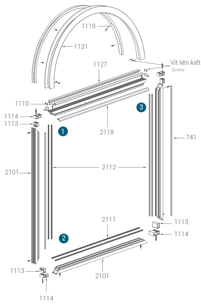
Chi tiết ráp khung bao Outer frame details
