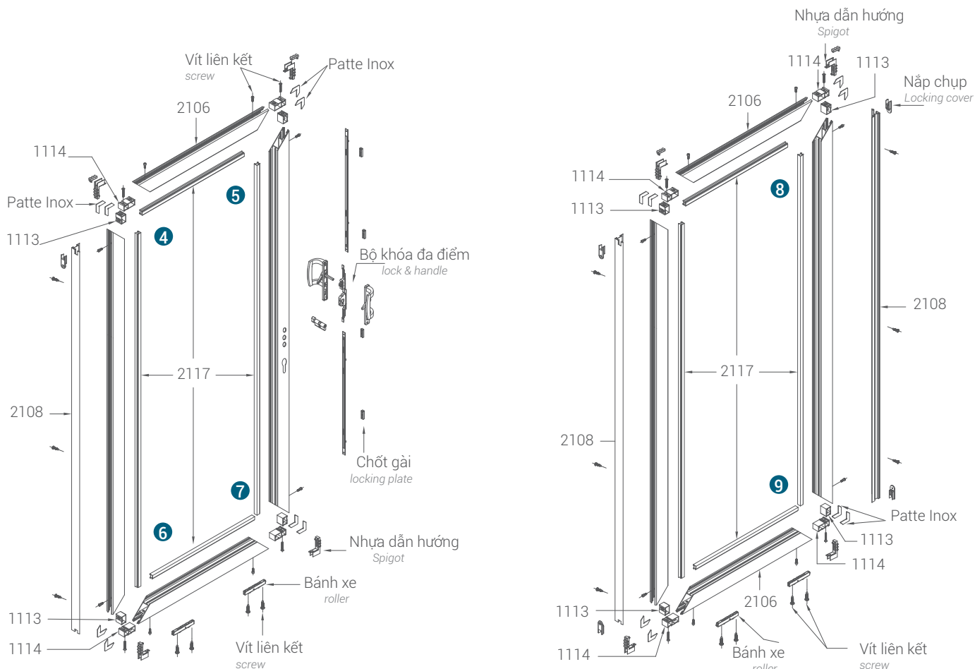
Chi tiết ráp khung cánh Leaf frame details
