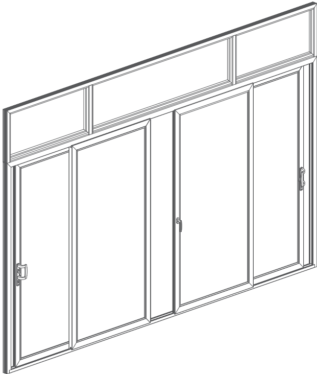
Lắp ráp hoàn thiện Complete assembly diagram
