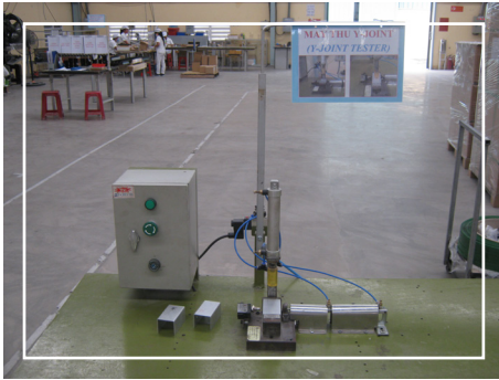
y-joint tester
